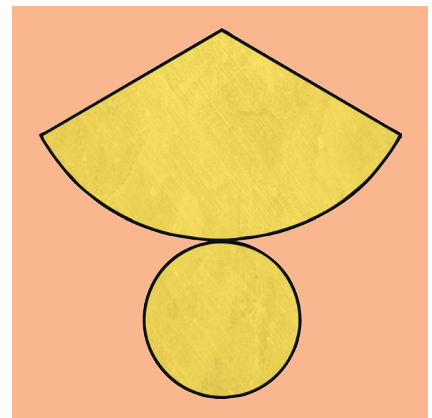
cone
